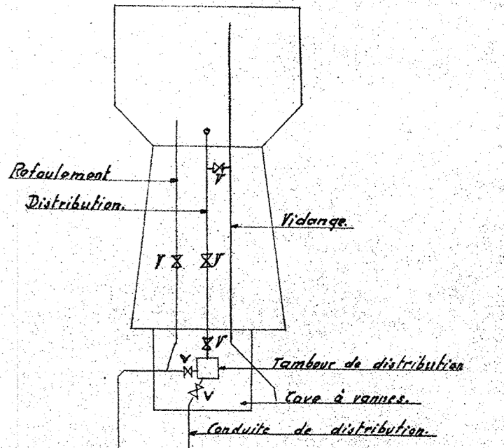
Détails du château d'eau.
