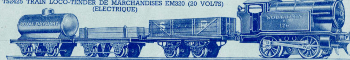
Ce Train est composé d'une Loco-Tender EM320 (avec renv. de marche commandé de la cabine et munie d'une Fumée avant), d'un Wagon de Marchandises, d'un Wagon à Bois de Charpente, d'un Wagon à Huile, et d'un jeu de rails électriques demandant une surface de 1 m. x 0 m. 75. Une Plaque de Connexion sert à relier la source de courant (Transformateur de 20 volts) à la voie.
