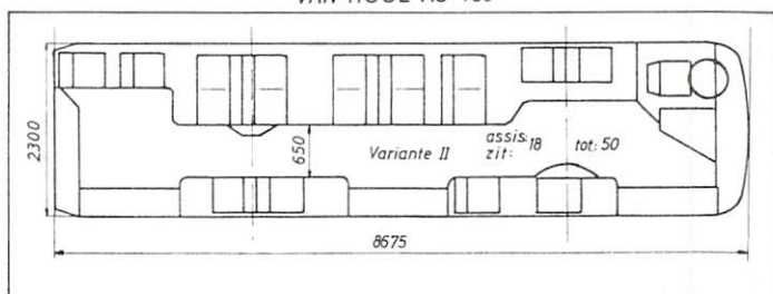
VAN HOOL AU 138
