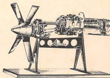
ALLISON TURBO-PROP MOTOR Opengewerkt beweegbaar model van de bekende vliegtuigmotor. Meerkleurig plastic, op standaard. H-1551 . . . . . f 31,50 H-1552 met elektro-aandrijving . . . . . f 37,95
