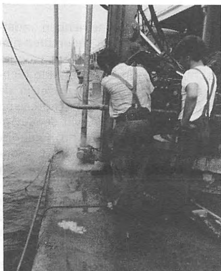
Met een zware drillboor worden hier op de kademuur de verticale ankerboringen geboord.
